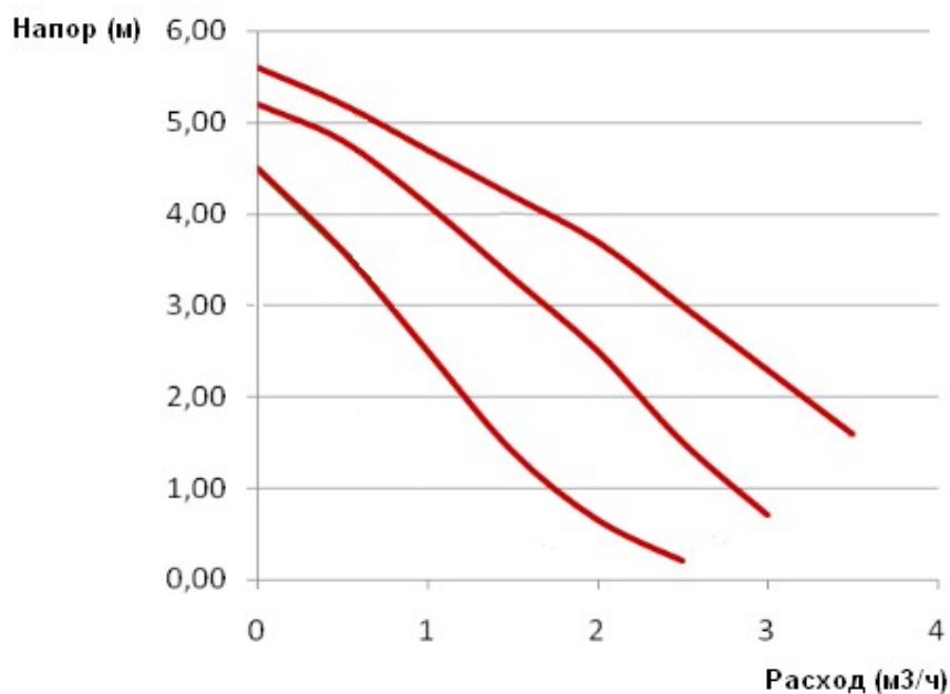
Grundfos UPSO 25-55
